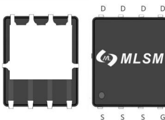
PDFN5X6-8L
