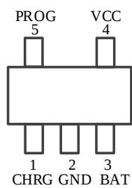
引脚信息
