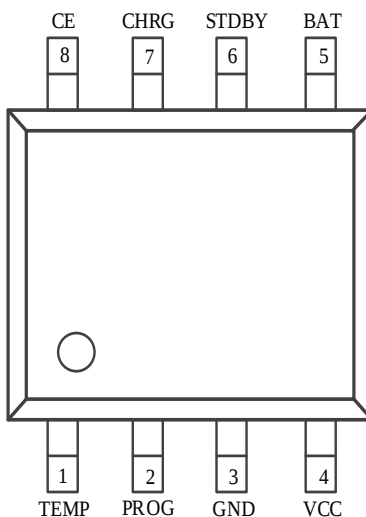
ESOP-8封装，散热片接地
