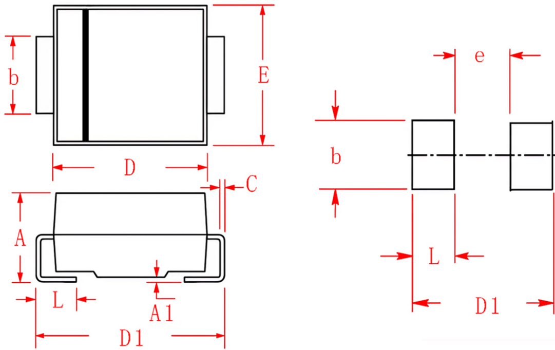
SMB (DO-214AA)
